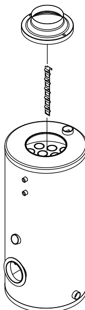
Рисунок 25. Схема доступа к жаротрубным каналам
