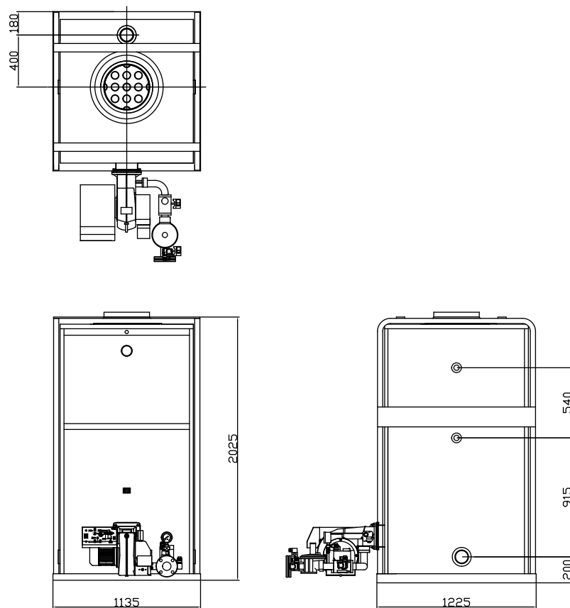
Рисунок 23. Габаритные и присоединительные размеры котлов KSG-400
